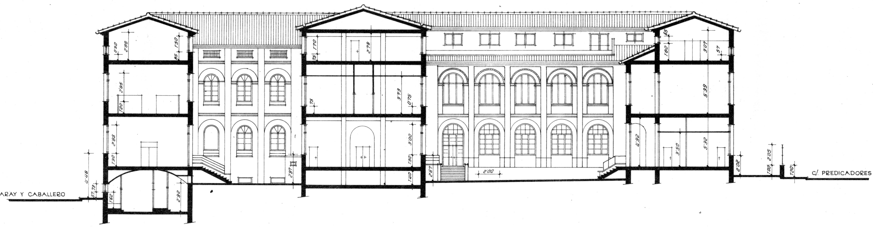
SECCION C - D
