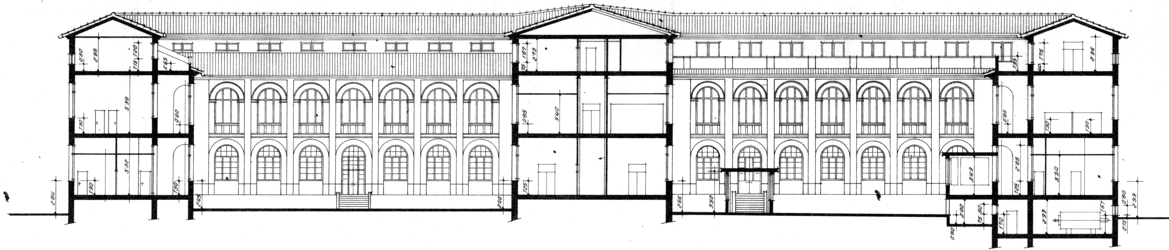
SECCION A - B
