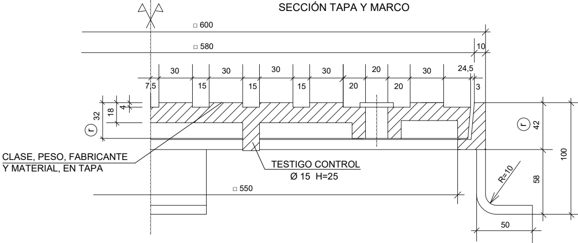
SECCIÓN TAPA Y MARCO
