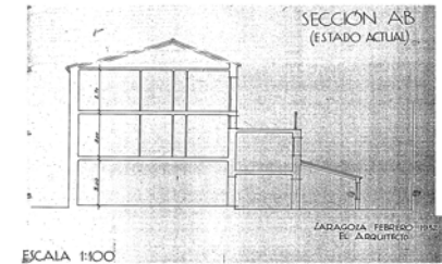
ESCALA 1:100
