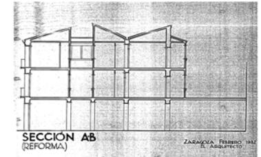
ESCALA 1:100
